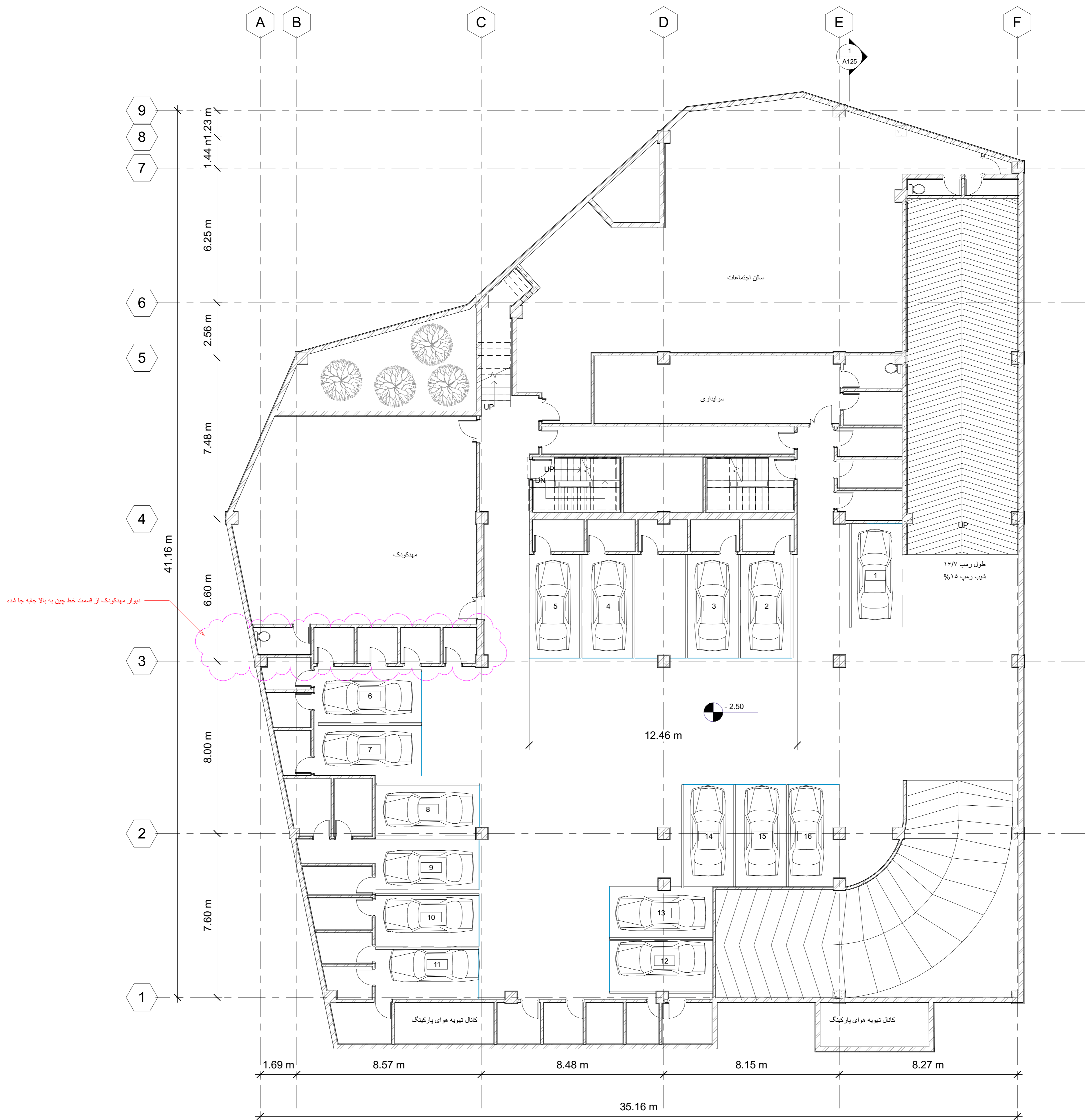
1 پلان زیرزمین اول. 08. 1 : 100
